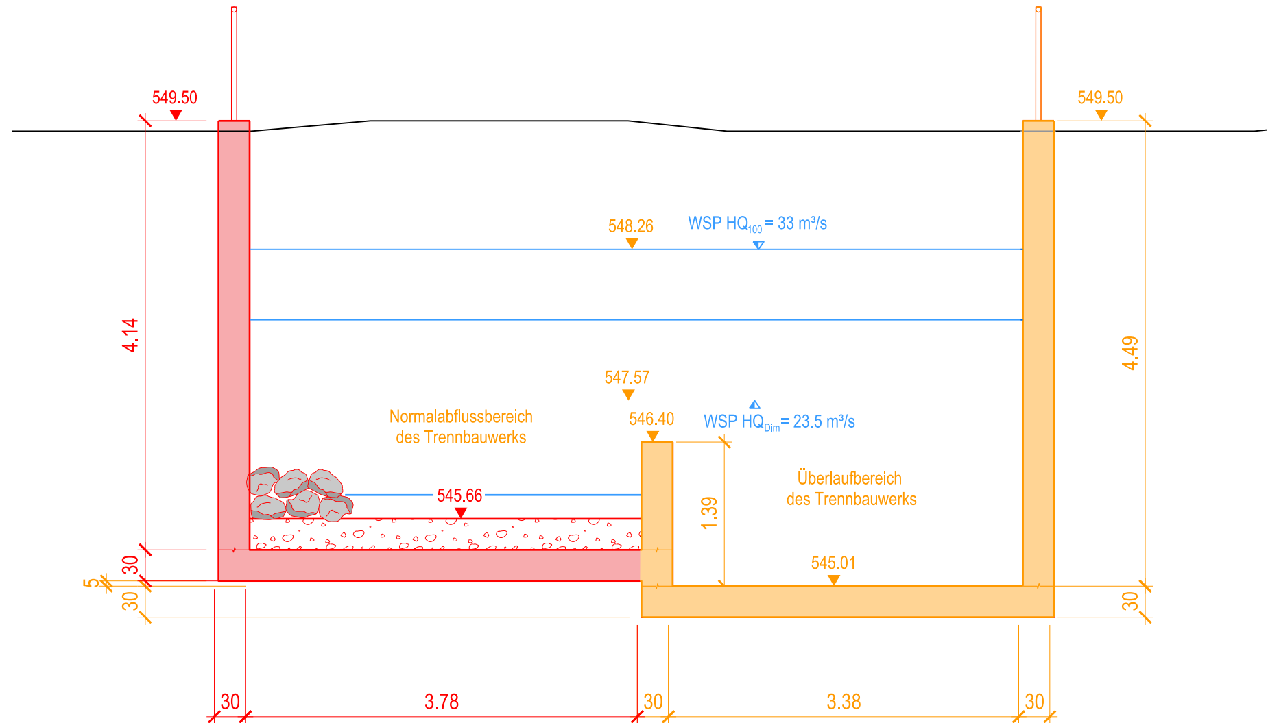
Überfallbauwerk zu Entlastungskanal
